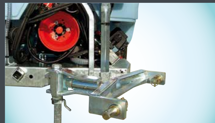
Timone articolato con cuscinetti / Tracker drawbar with bearings / Attelage articulé avec roulements / Gelenkdeichsel mit Lager / Tiro articulado con cojinetes
