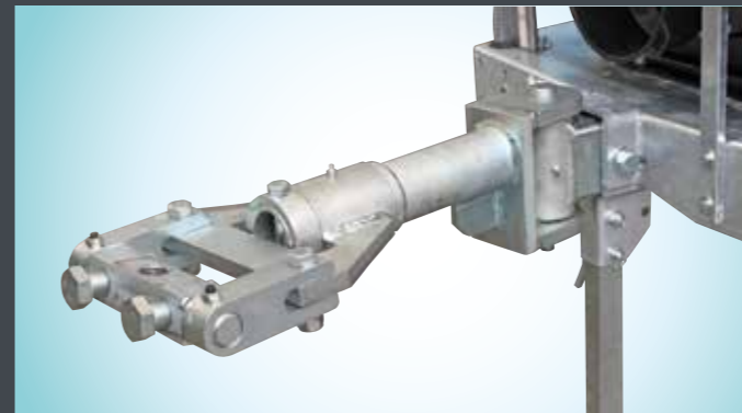
Timone sterzante con cuscinetti tipo Germania / Tracker drawbar with bearings "German type" / Attelage articulé monté sur roulement modèle Germania / Lenkdeichseln mit Lager Germania Modell / Tiro articulado con cojinetes tipo Alemania
